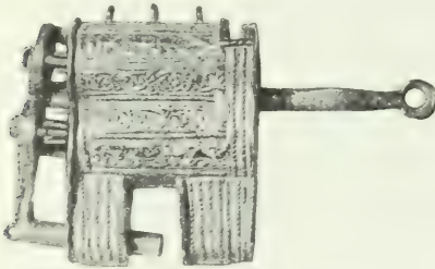
Hængelaas fra det 12te—13de Aarhundrede. Nøglen sidder i. Laasen aabnes ikke ved, at Nøglen drejes om, men ved at Bundstykket og Bolten — som vist — stødes ud med Nøglen.
